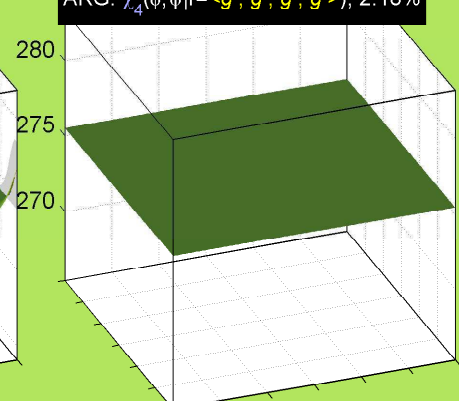
ARG: \chi_4(\phi, \psi | r = \langle g^-, g^-, g^-, g^- \rangle) , 2.18%
